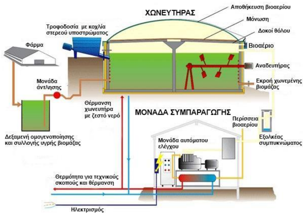
Εικόνα 6. Στάδια λειτουργίας μονάδας βιοαερίου
